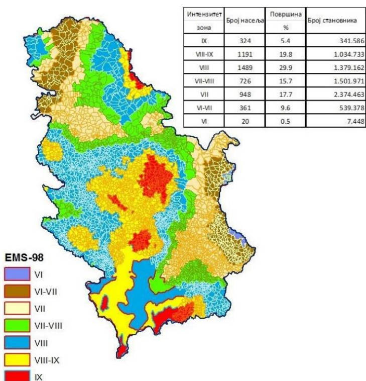
Слика 2. Преглед интензитета земљотреса и броја становника на одређеним подручјима (Ministarstvo unutrašnjih poslova R. Srbije, 2017)
