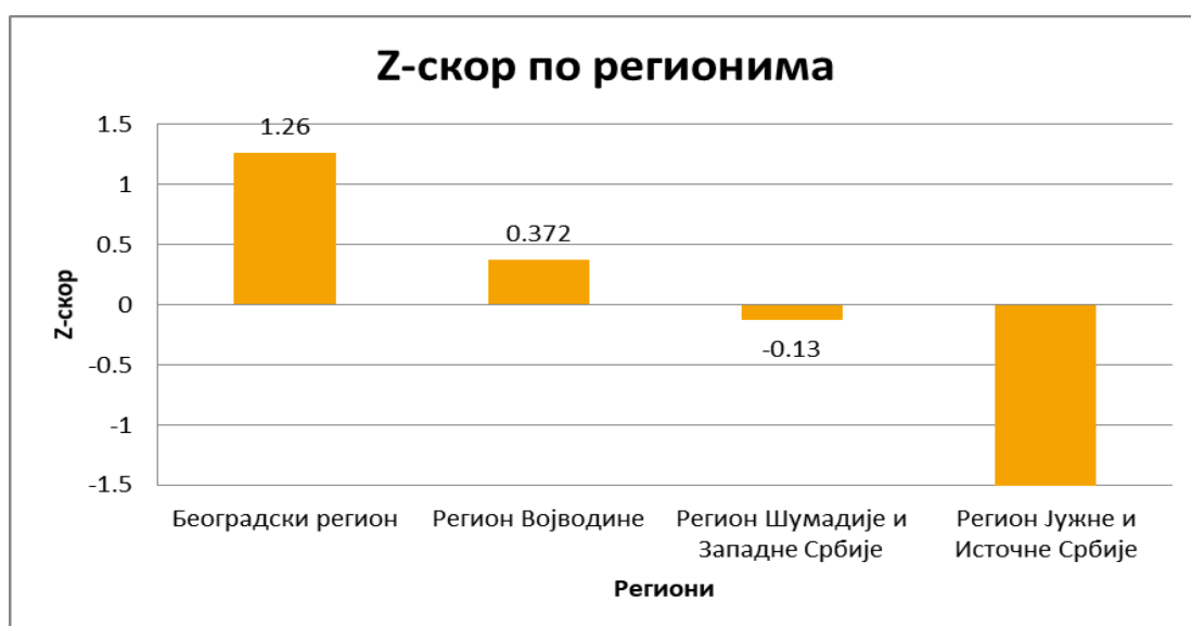
Графикон 2. BRIC Z-скорови по регионима. Z = (x - \mu) / \sigma , где су \mu 0.4918 и \sigma = 0.0518 (рачунато преко наведених региона). Позитиван Z означава изнадпросечну отпорност, негативан испод просечну; испрекидана нулта линија представља просек.
